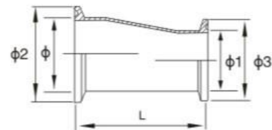
(偏心Eccentric)
