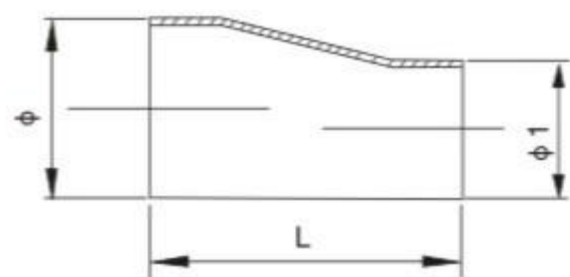
(偏心 Eccentric)
